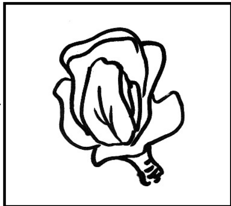
4. head fattens
